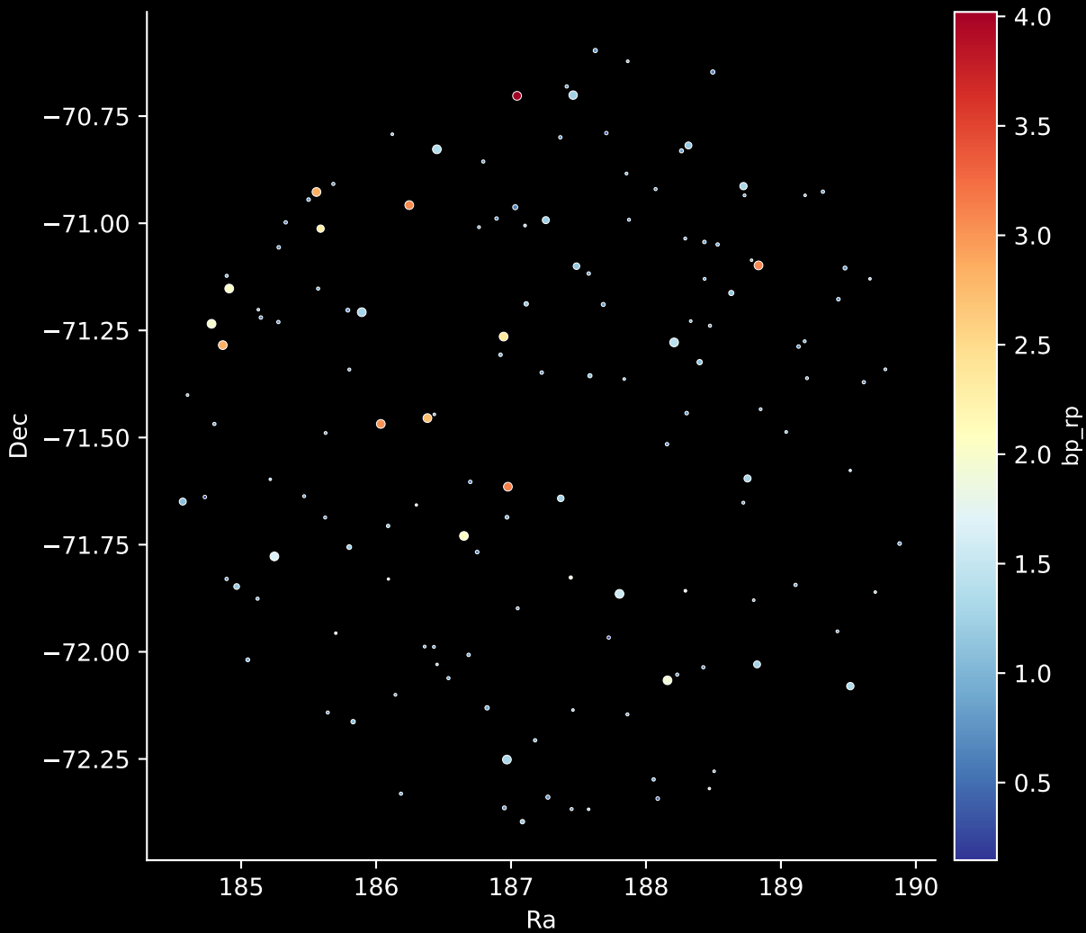
APOGEE DR17 Field: [282-31-O_TESS] Stars: 143
