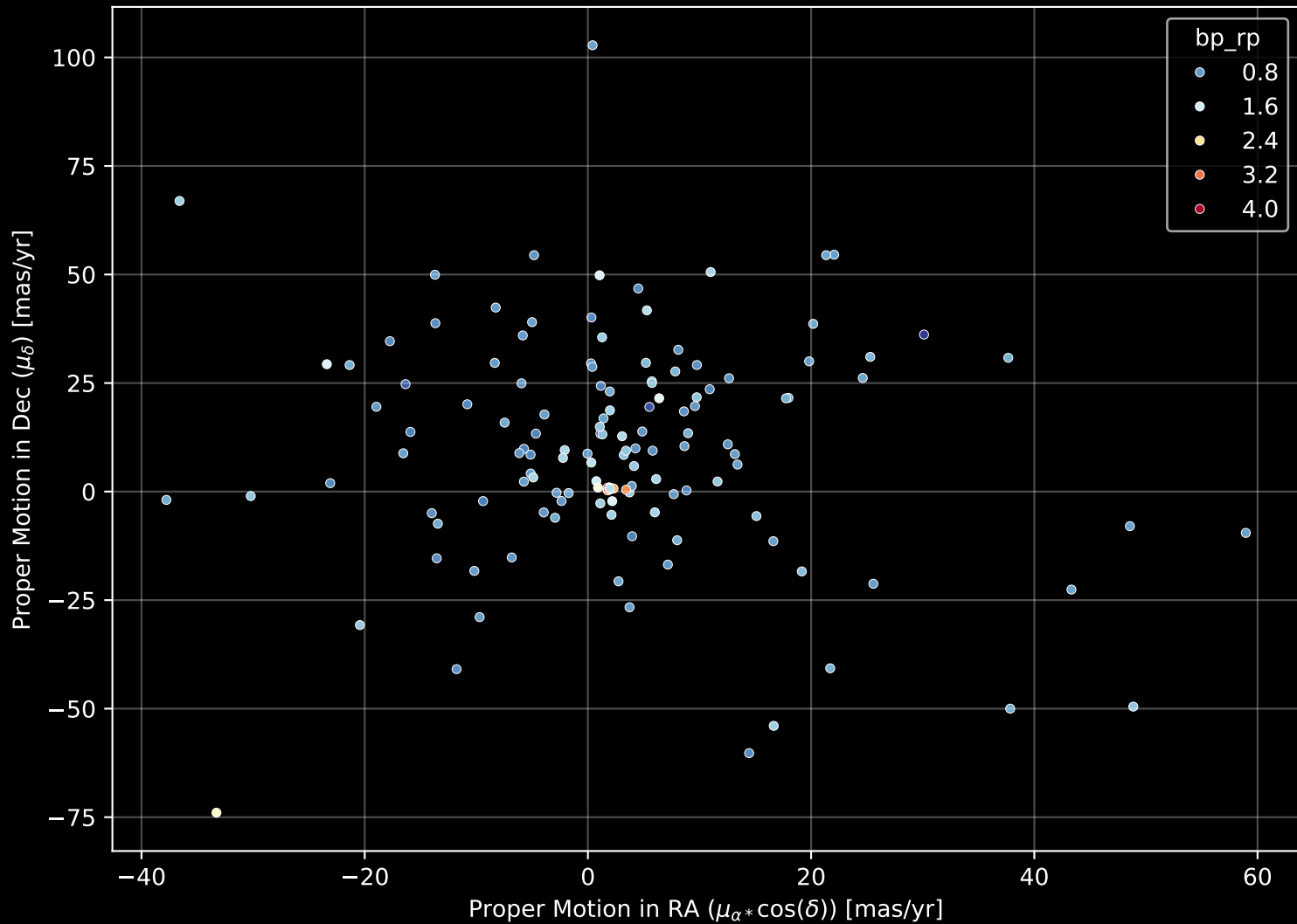
APOGEE DR17 Field: [282-31-O_TESS] Proper Motion Diagram (n= 143)
