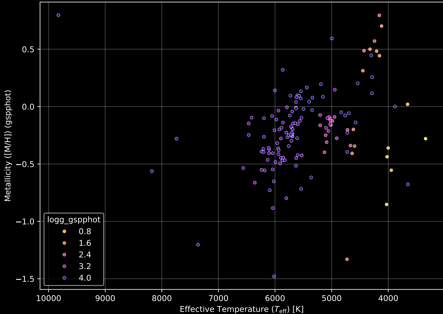
APOGEE DR17 Field: [282-31-O_TESS] Stellar Population Parameters (n= 143)
