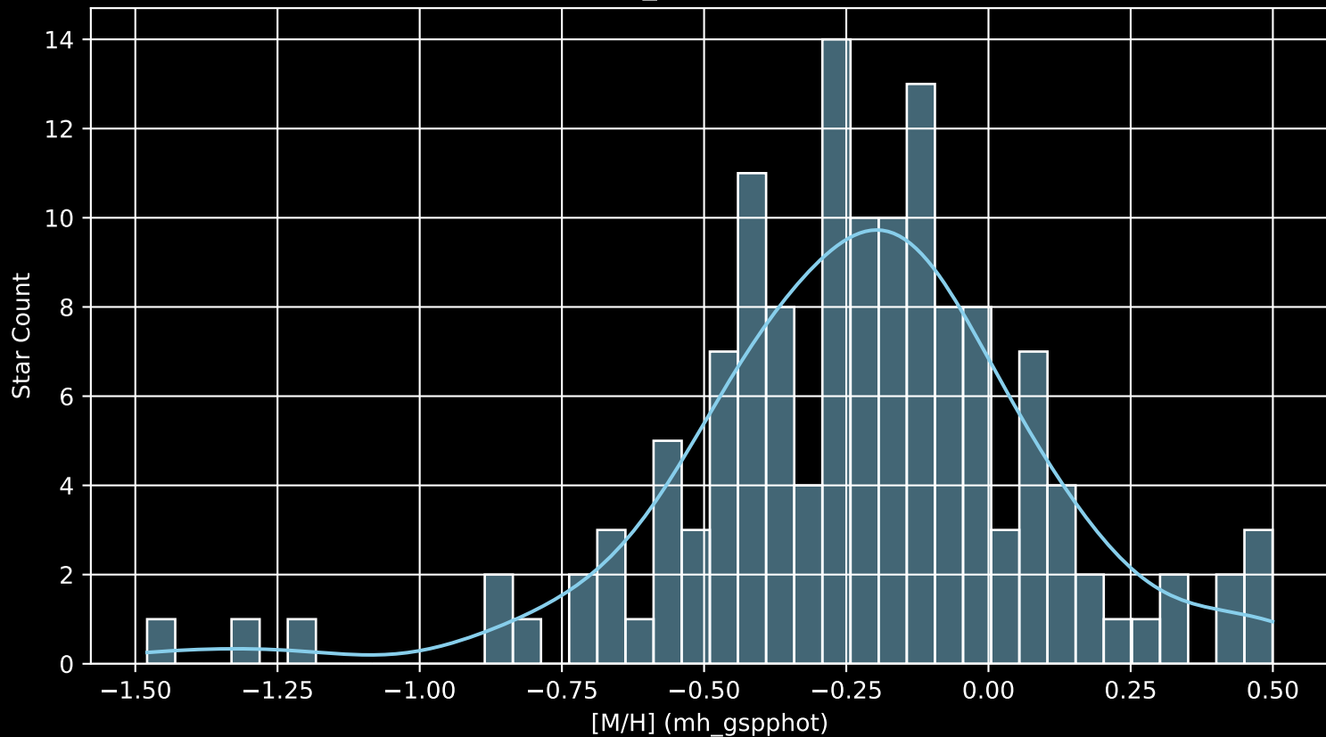
APOGEE DR17 Field: [282-31-O_TESS [M/H] (mh_gspphot) (n= 138)
