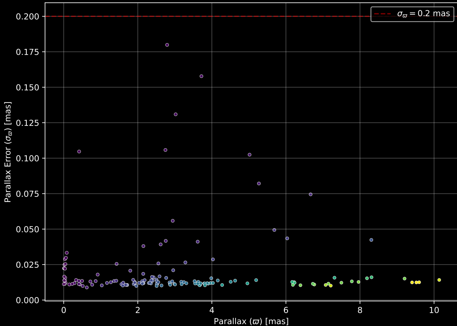
APOGEE DR17 Field: [282-31-O_TESS] Parallax Quality (n= 143)
